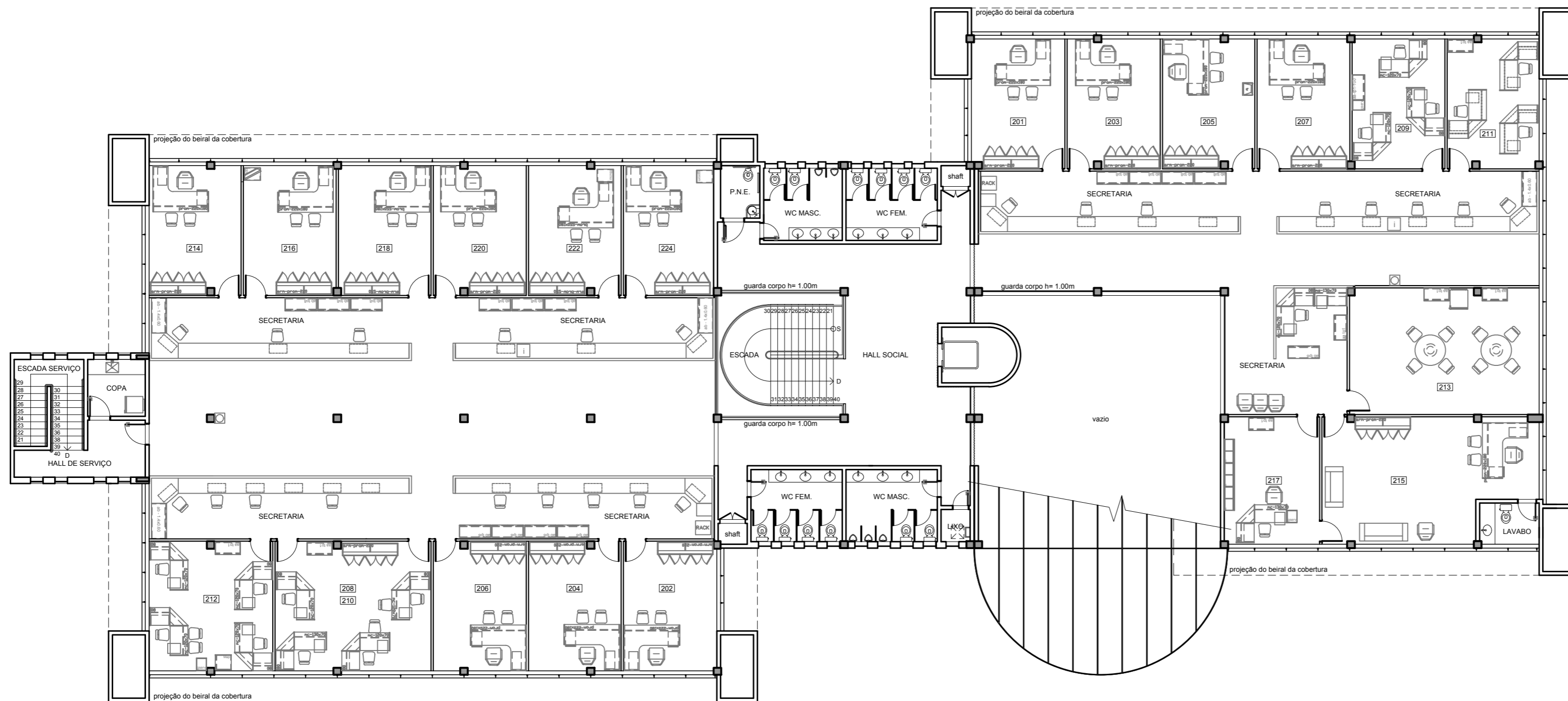
LAYOUT - 1º PAVIMENTO esc 1/100
